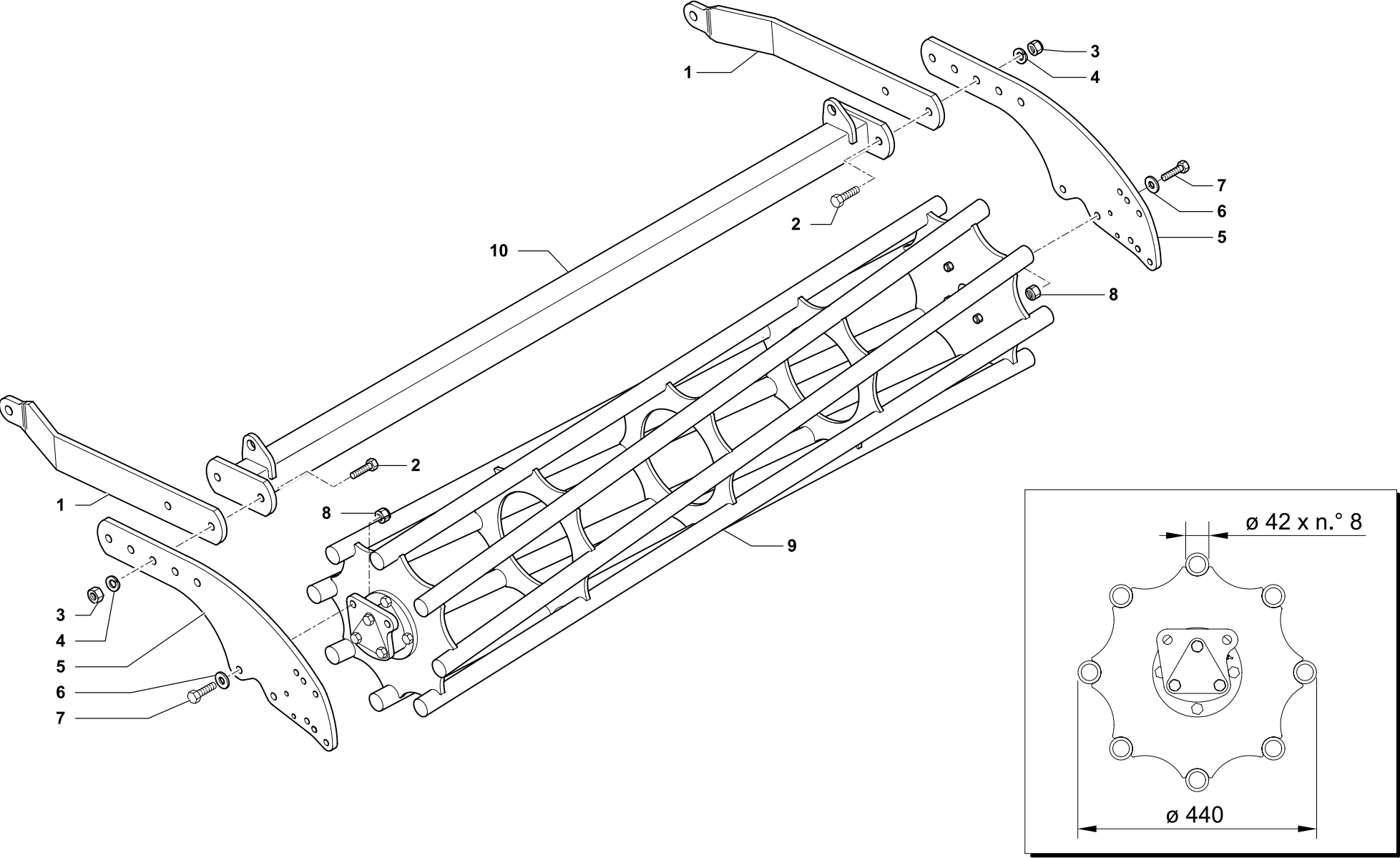
CAGE ROLLER Ø 440
