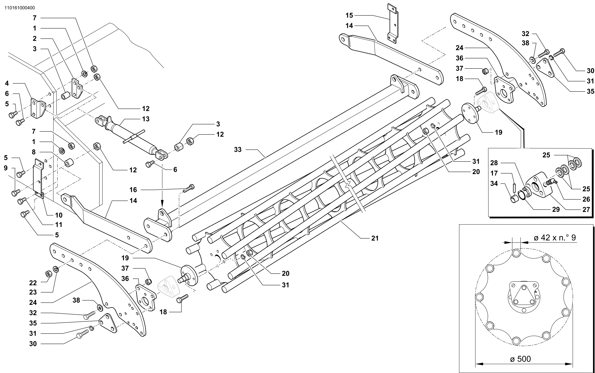
CAGE ROLLER Ø 500
